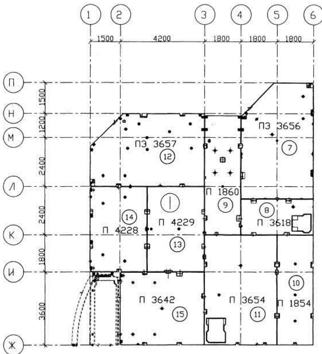
Рис. 4. Схема монтажа перекрытия этажа
