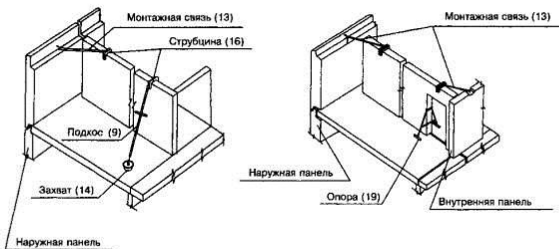
Рис. 2 Типовое крепление сборных элементов
