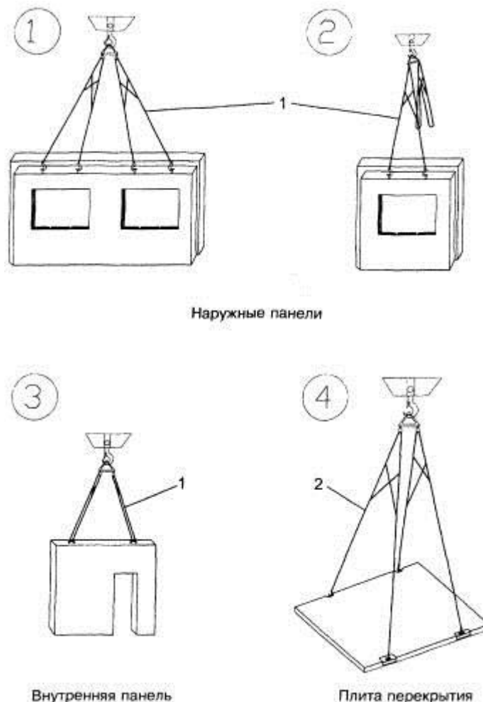
Рис. 1. Схемы строповки
