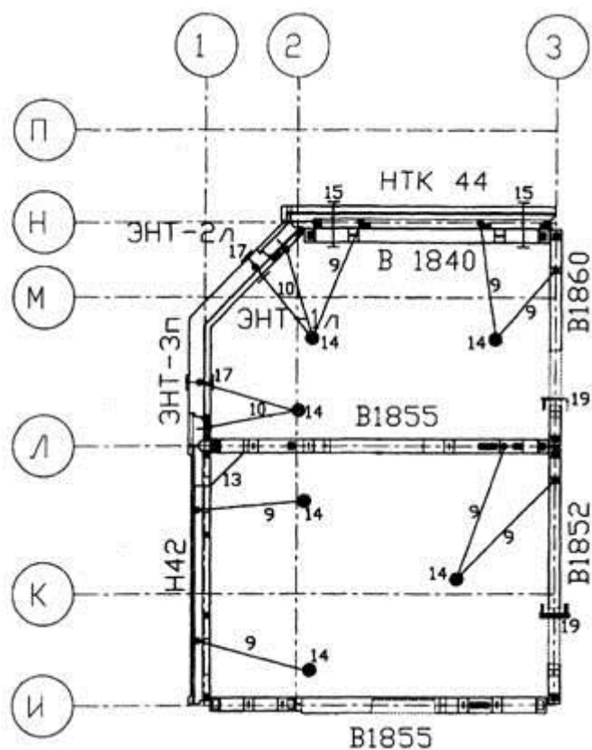
Рис. 8. Схема временного крепления сборных элементов
