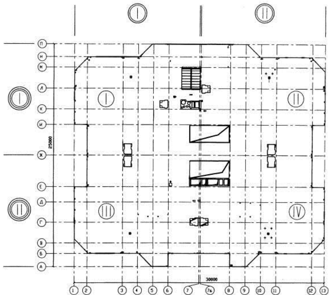
Рис. 3. Варианты деления на захватки этажа дома
