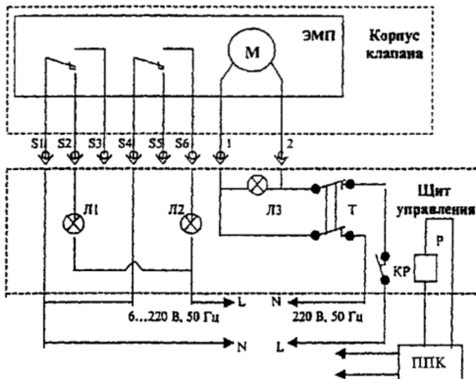
Электрическая схема подключения клапана КДМ-2 с приводом «Velimo»
