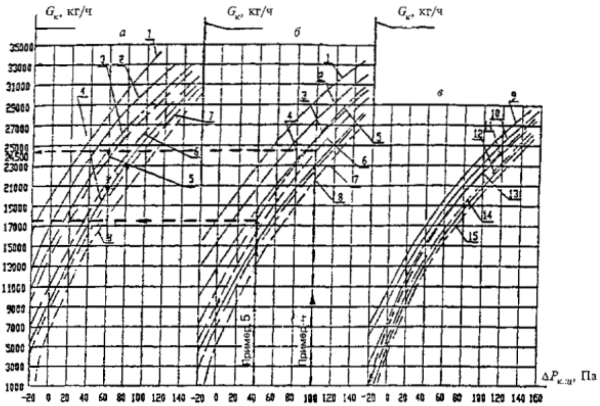
Рис. 4. Планировка Б. Расход воздуха G_k , кг/ч, для незадымляемой лестничной клетки 2-го типа в зависимости от разности давлений между лестничной клеткой и лифтовой шахтой \Delta P_{k.ш} , Па, на верхнем этаже и от давления в лифтовой шахте на 1-м этаже P_{ш1} , Па
