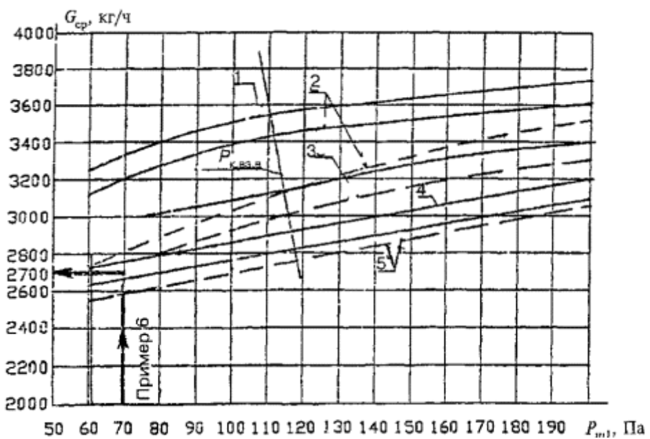
Рис. 8. Планировка В. Средний расход наружного воздуха, кг/ч, для верхней зоны здания из 5 или 13 этажей с внутренним переходом в нижнюю зону в зависимости от давления воздуха в лифтовой
