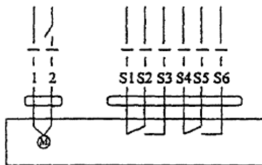
Контактная группа
