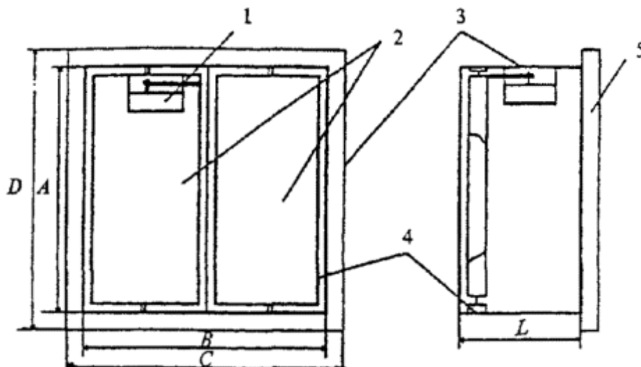
Стеновой дымовой клапан
