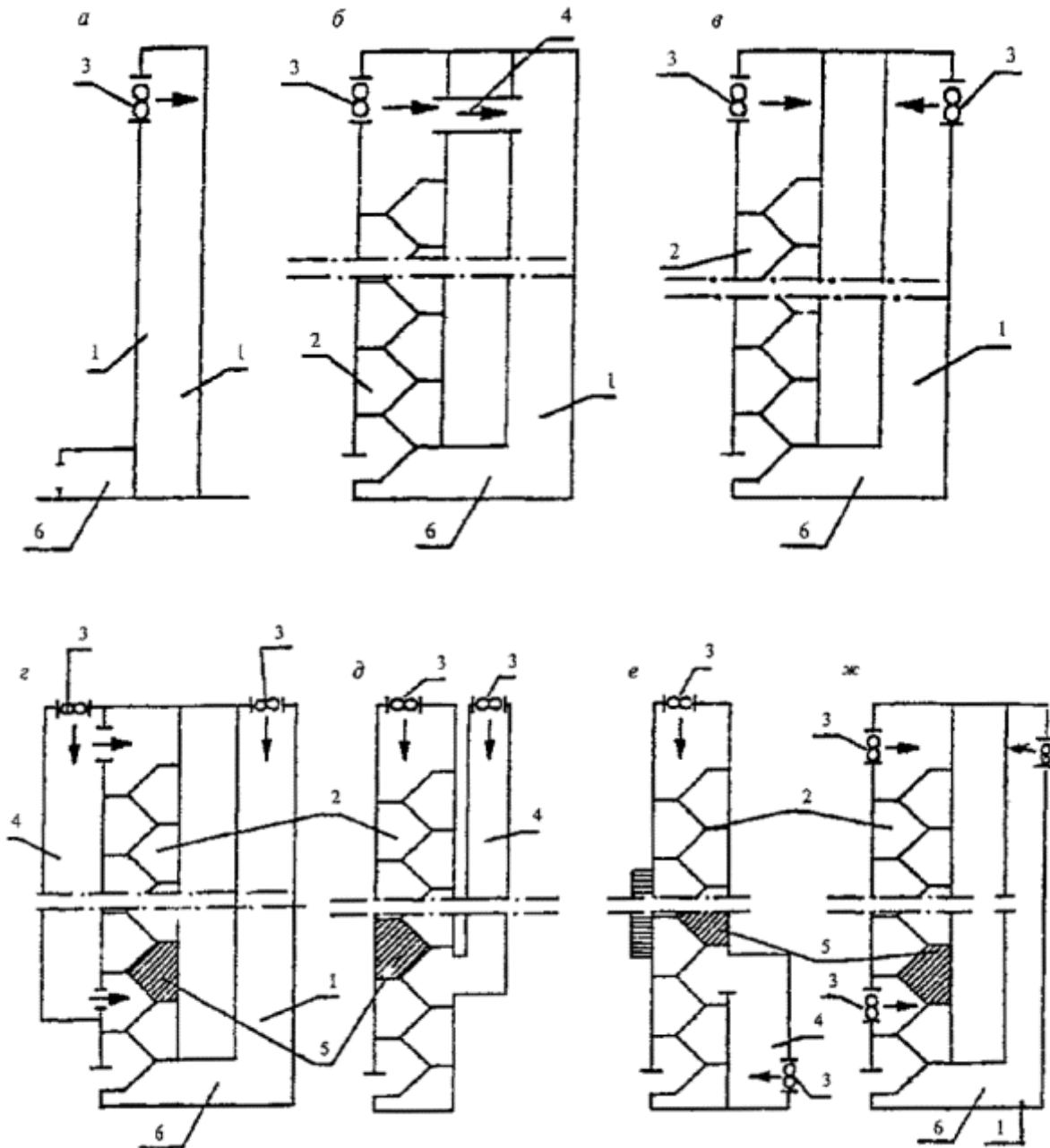
Рис. 2. Принципиальные схемы подачи наружного воздуха в незадымляемые лестничные клетки 2-го типа и лифтовые шахты
