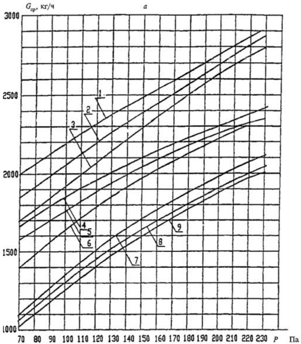
Рис. 3. Средний расход воздуха G_{ср} , кг/ч, на каждый этаж со 2-го по верхний в зависимости от давления воздуха в лифтовой шахте на 1-м этаже P_{ш1} , Па, числа дверей на этаже и температуры наружного воздуха в холодный период года (параметры Б) для 1-14-этажного (а), для 15-20-этажного (б) и 21-27-этажного (в) здания
