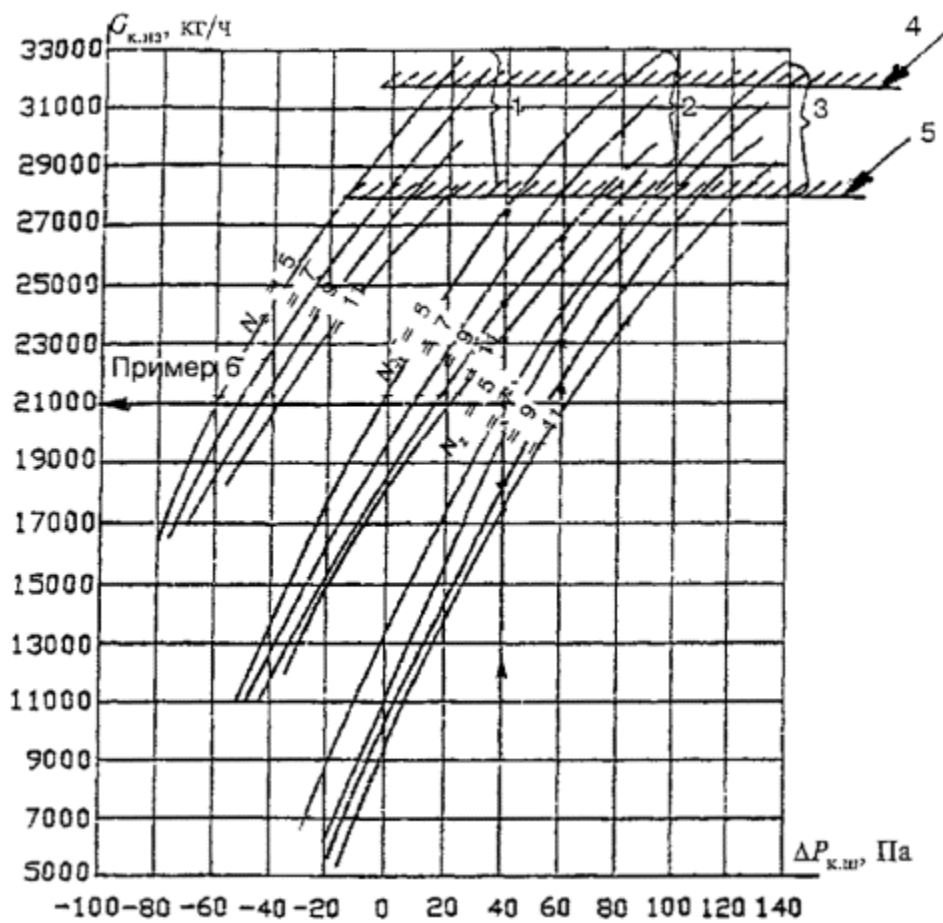
Рис. 7. Планировка В. Расход наружного воздуха G_{к,кг} , кг/ч, в нижнюю зону лестничной клетки 2-го типа при P_{ш1} , равном 1 - 190 Па; 2 - 110 Па; 5 - 30 Па; 4 - предельный расход воздуха при 7 этажах в зоне; 5 - то же, при 11 этажах в зоне с внутренним переходом между зонами; 7 - число этажей
