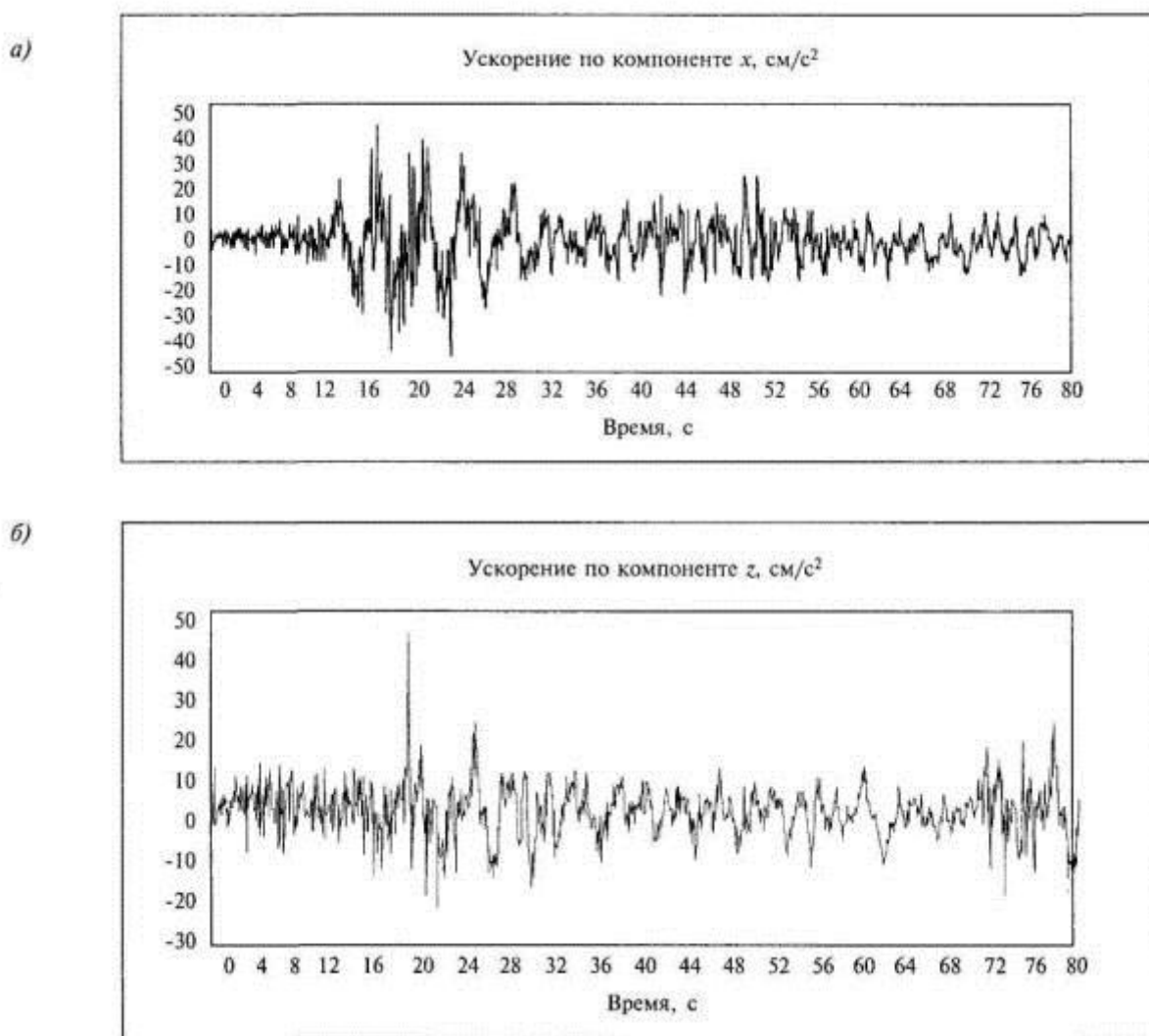
Рисунок 7.1. Акселерограммы землетрясения 4 марта 1977 г., зарегистрированные на расстоянии 1400 км от эпицентра (Москва находится на таком же расстоянии от зоны Вранчских очагов) a) - компонента x; б) - компонента z
