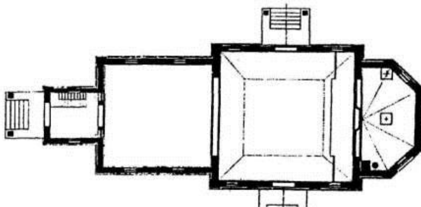
Проект деревянной церкви на 400-500 чел.
