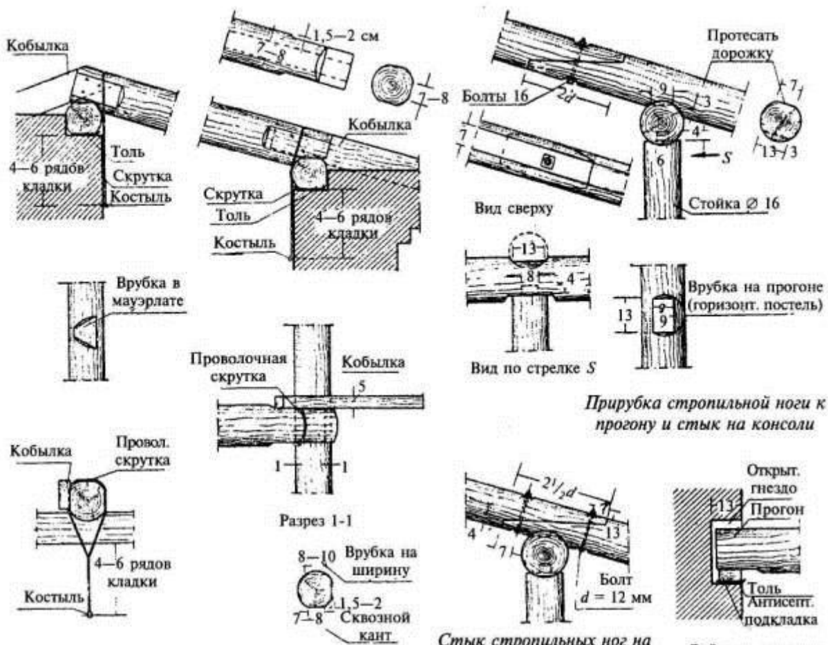
Заделка прогона в стену
