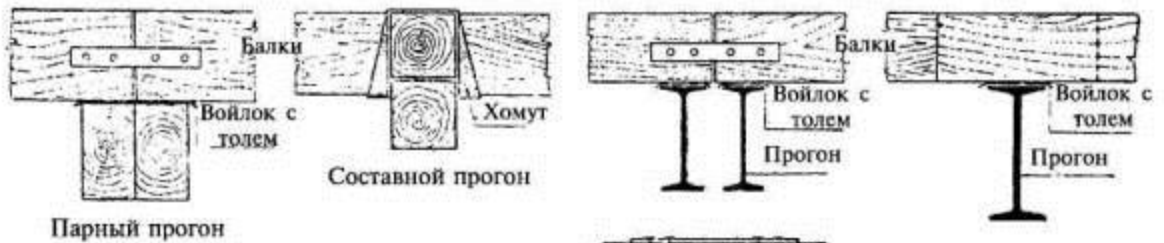
Опирающие прогоны
