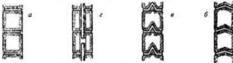
Сплачивание венцов из брусьев
