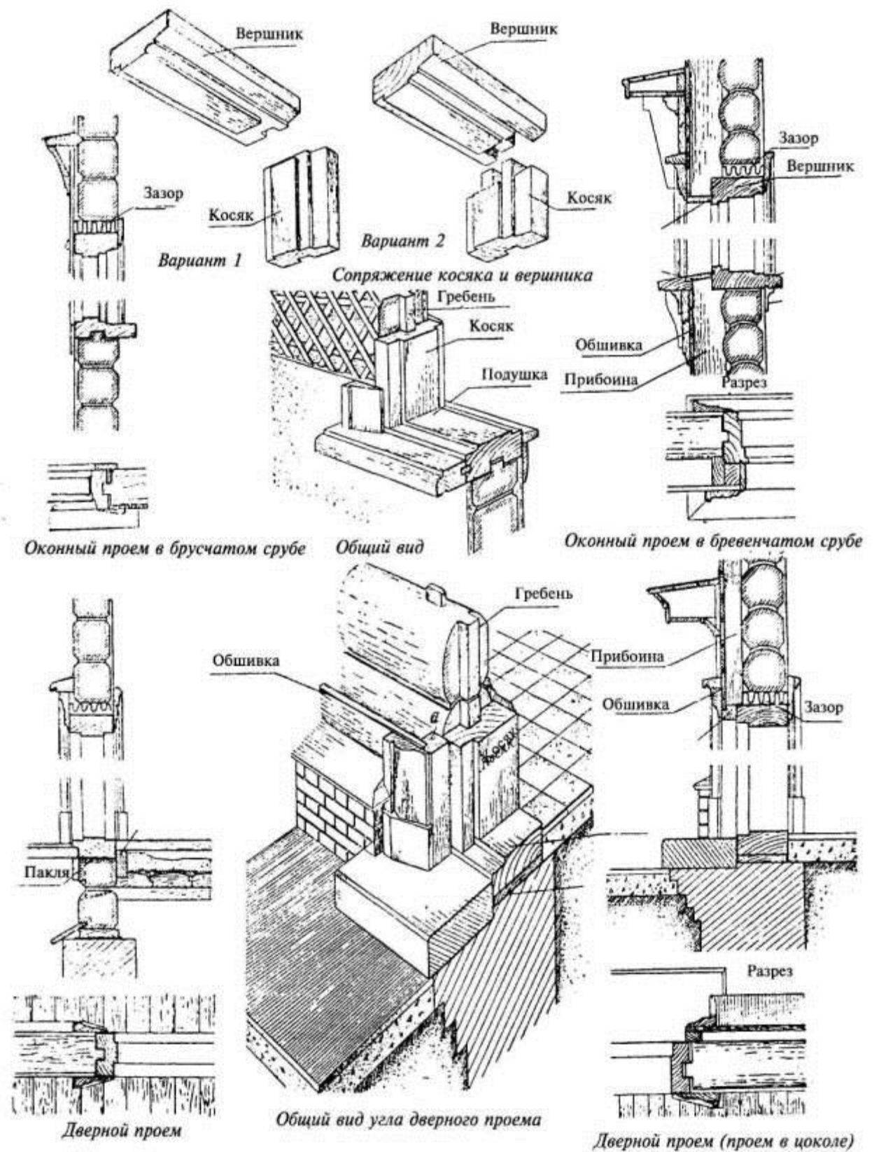
Обделка оконных и дверных проемов
