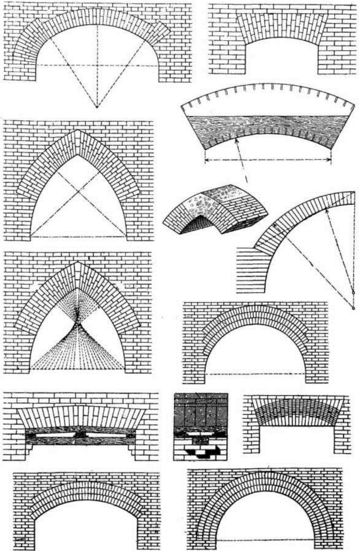
Арки и своды (из Руководства В.Р. Бернгарда, 1901)
