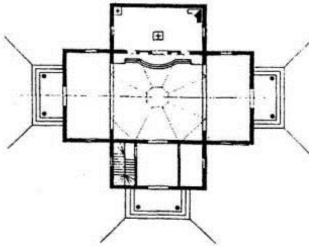
Проект деревянной церкви на 400 чел.
