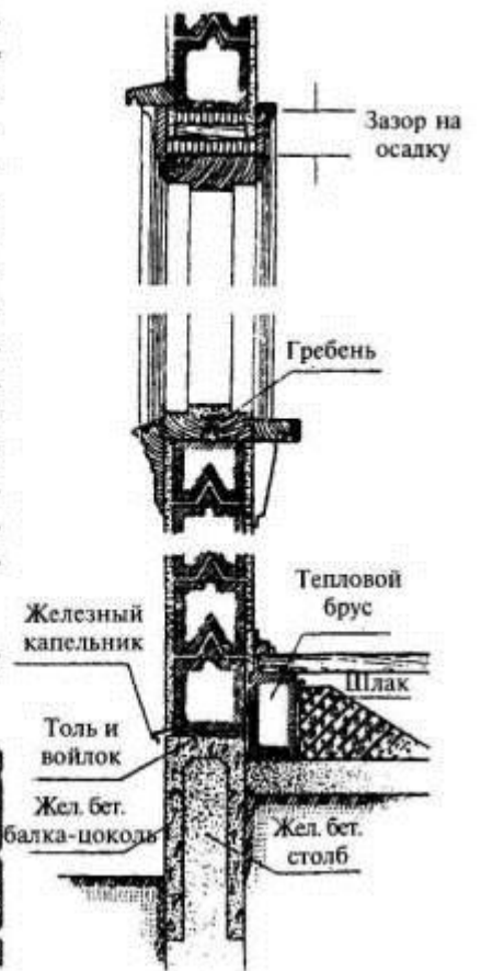
Стена из брусьев на сборном жел. бет. фундаменте
