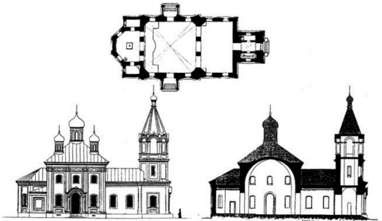
Проект каменной церкви на 500 чел. (1899)
