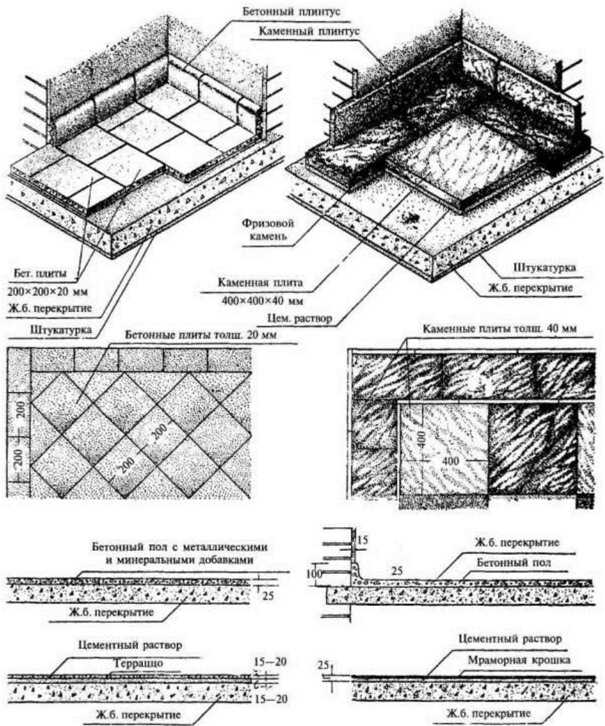
Полы из естественных камней и бетонные
