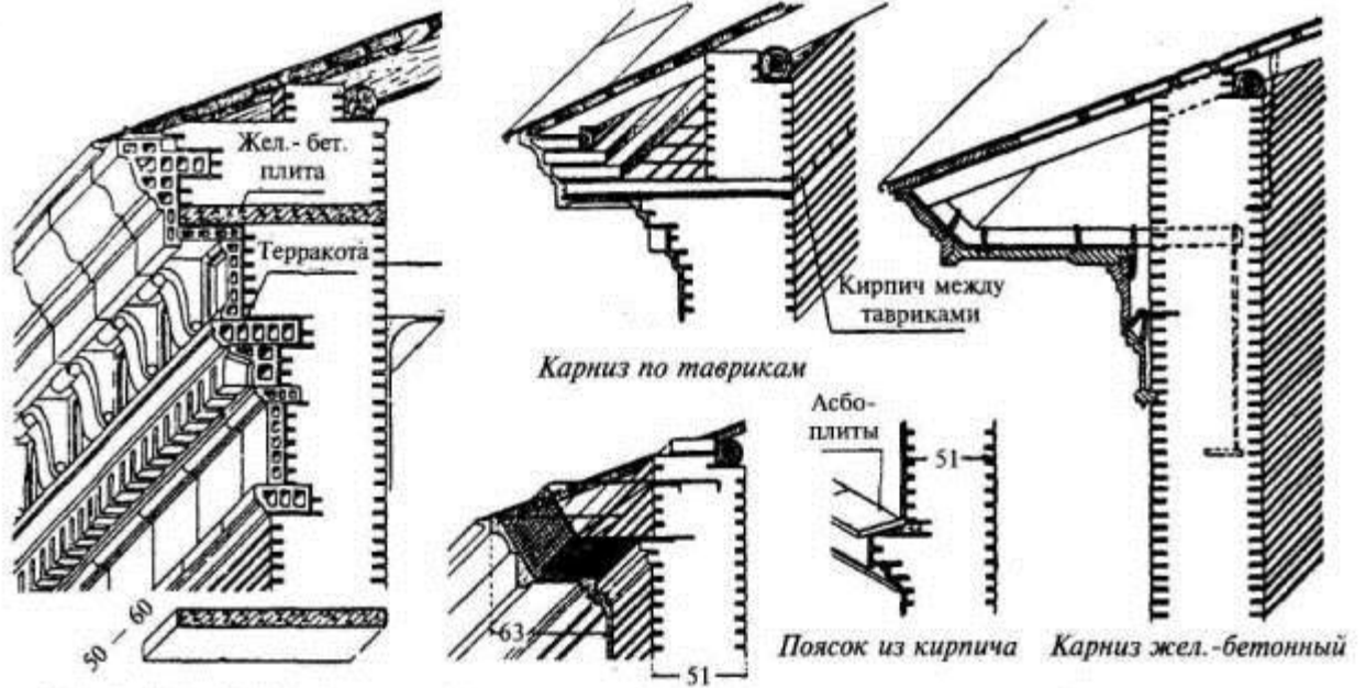
Карниз терракотовый
