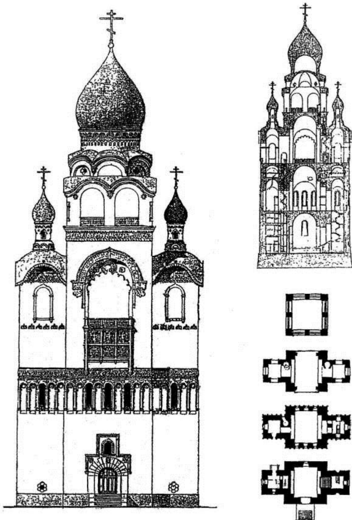
Архитектор Ф.Ф. Горностаев Конкурсный проект Воскресенского храма на Рогожском кладбище в Москве (1915)
