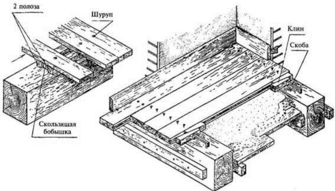
Полы дощатые, простые
