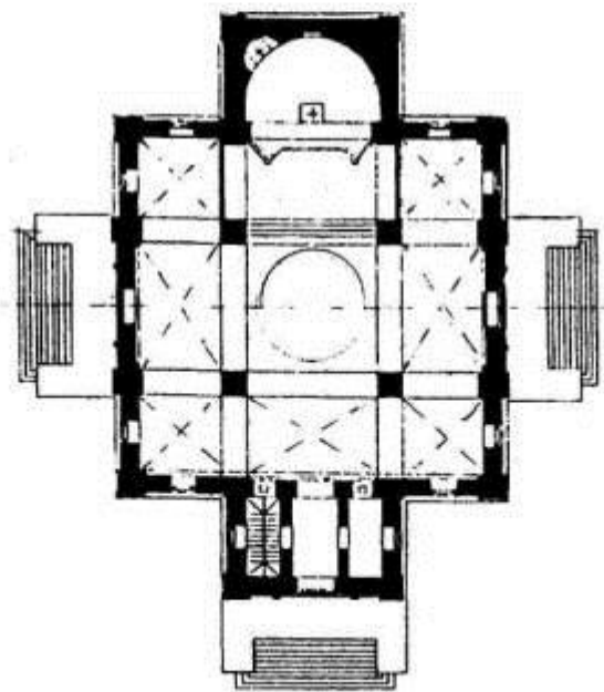
Проект каменной церкви на 750 чел. (1899)
