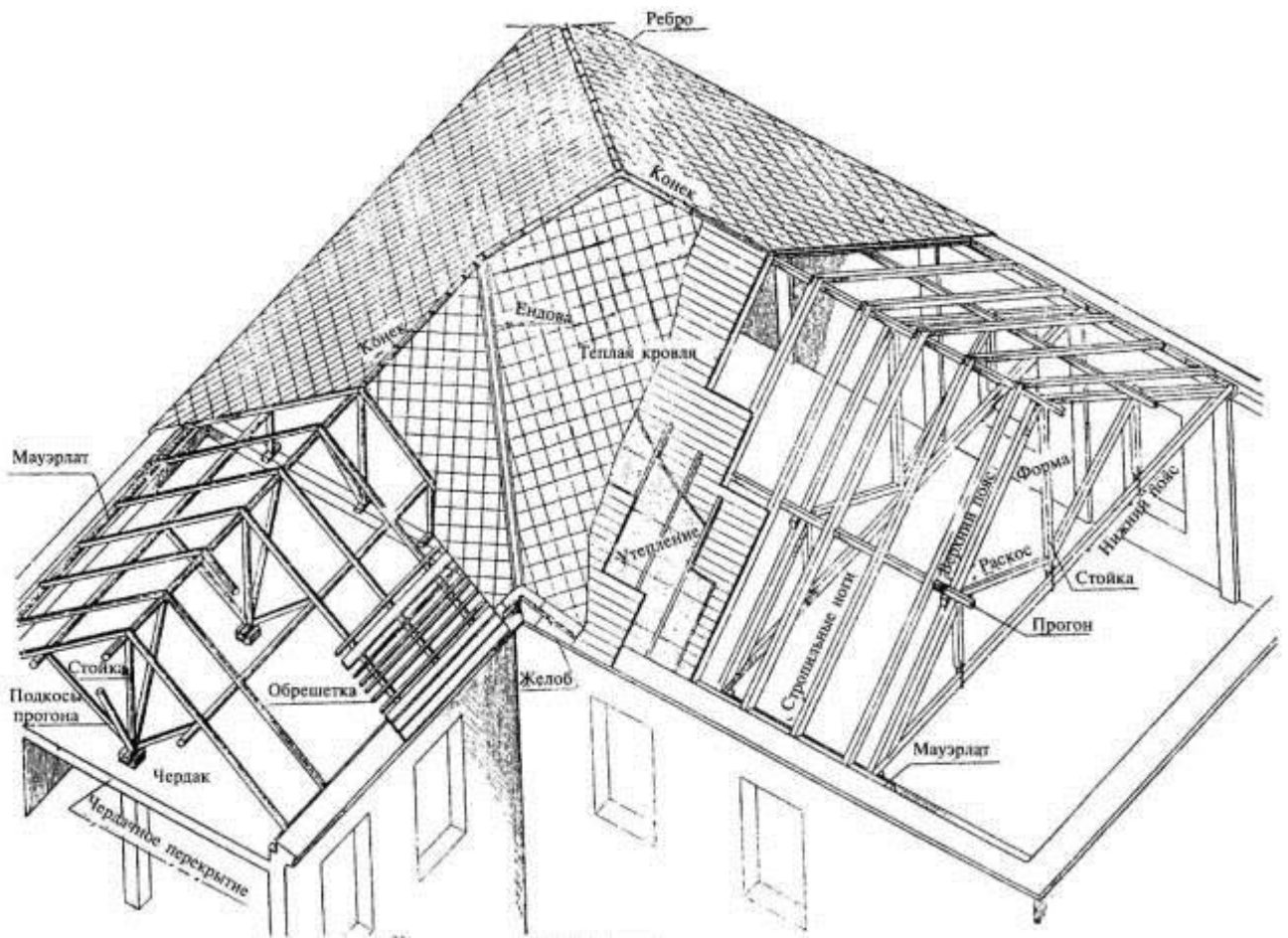
Конструкция крыши и ее элементы
