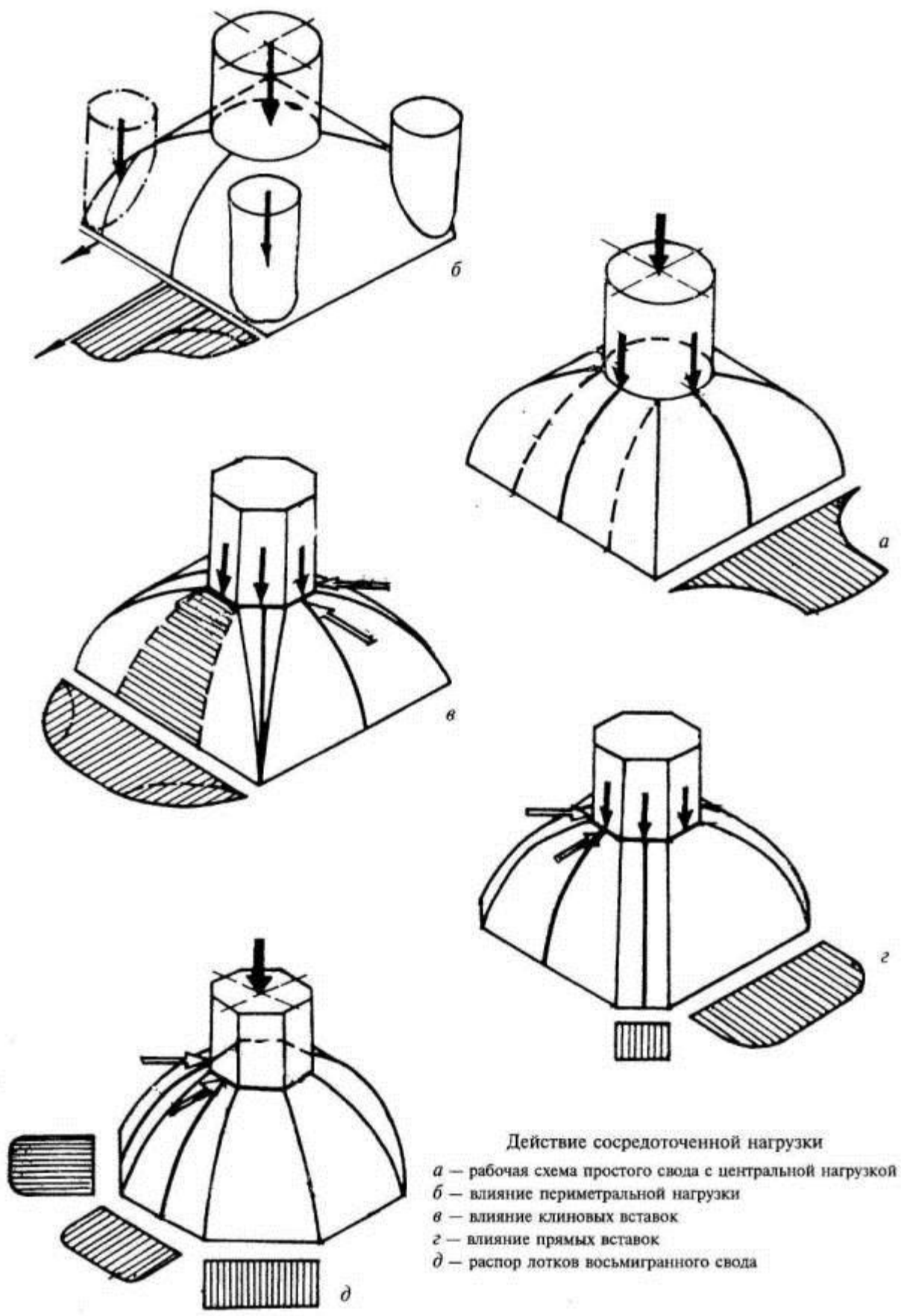
Своды (схема Г.В. Бессонова)
