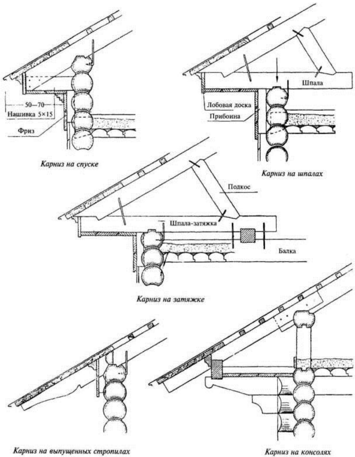
Конструкции карнизов рубленых домов
