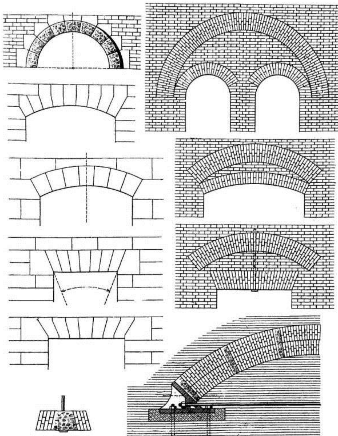
Арки и своды (из Руководства В.Р. Бернгарда, 1901)
