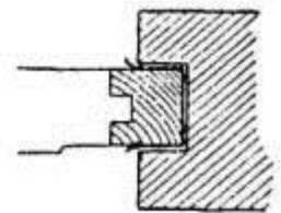
Присоединение рубленых стен к каменным
