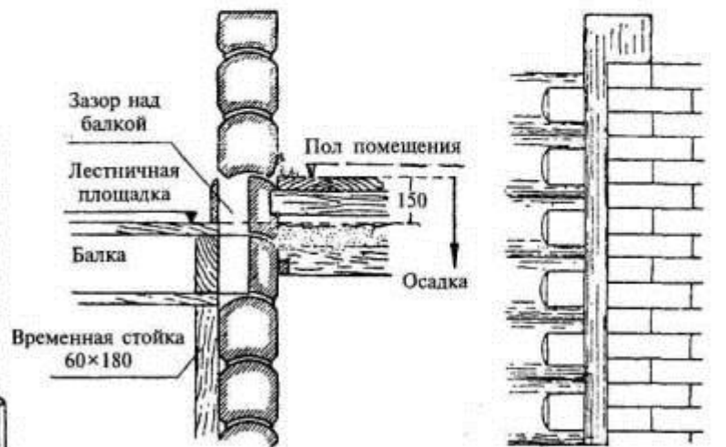
Присоединение лестничной площадки в 2-этажном здании
