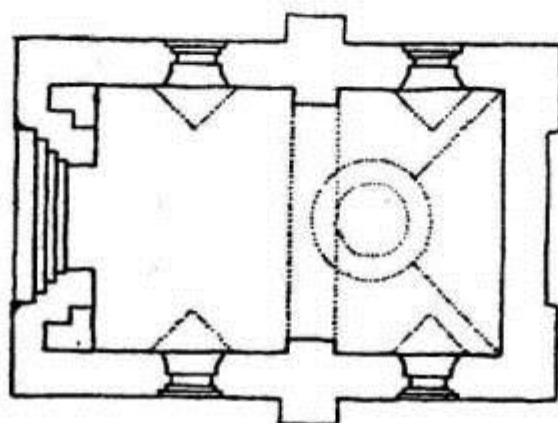
Архитектор М. Ерофеев Проект часовни при фабричной больнице т-ва Сапожниковых (1914)
