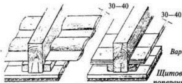
Накат из горбылей и досок
