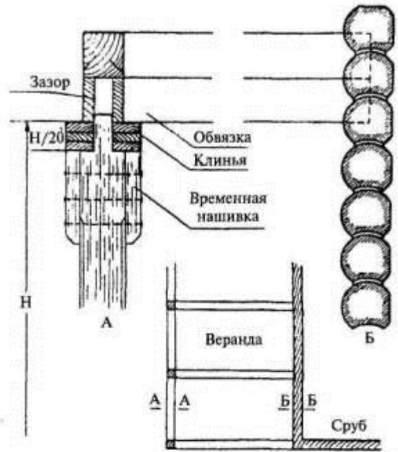
Соединение стоек веранды со стеной (Вариант II)
