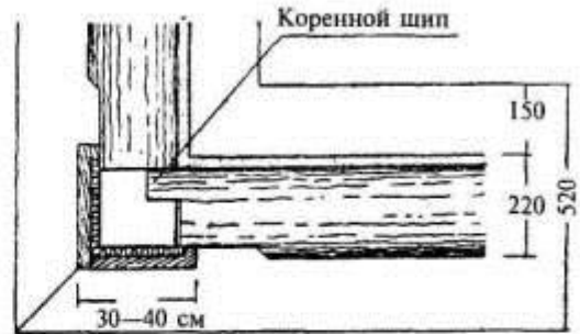
Сруб без остатка
