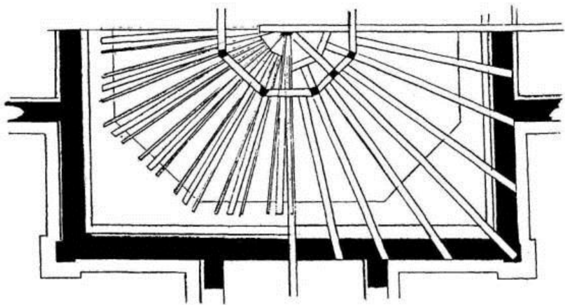
Конструкция деревянного покрытия храма (из атласа проектов храмов, 1911)
