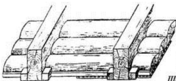
Накат подрезной из пластин
