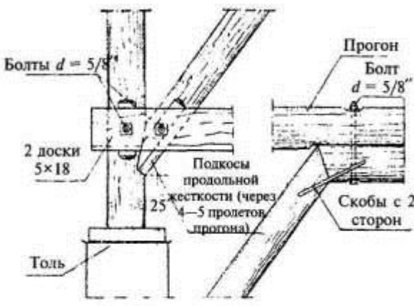
Детали шпренгеля
