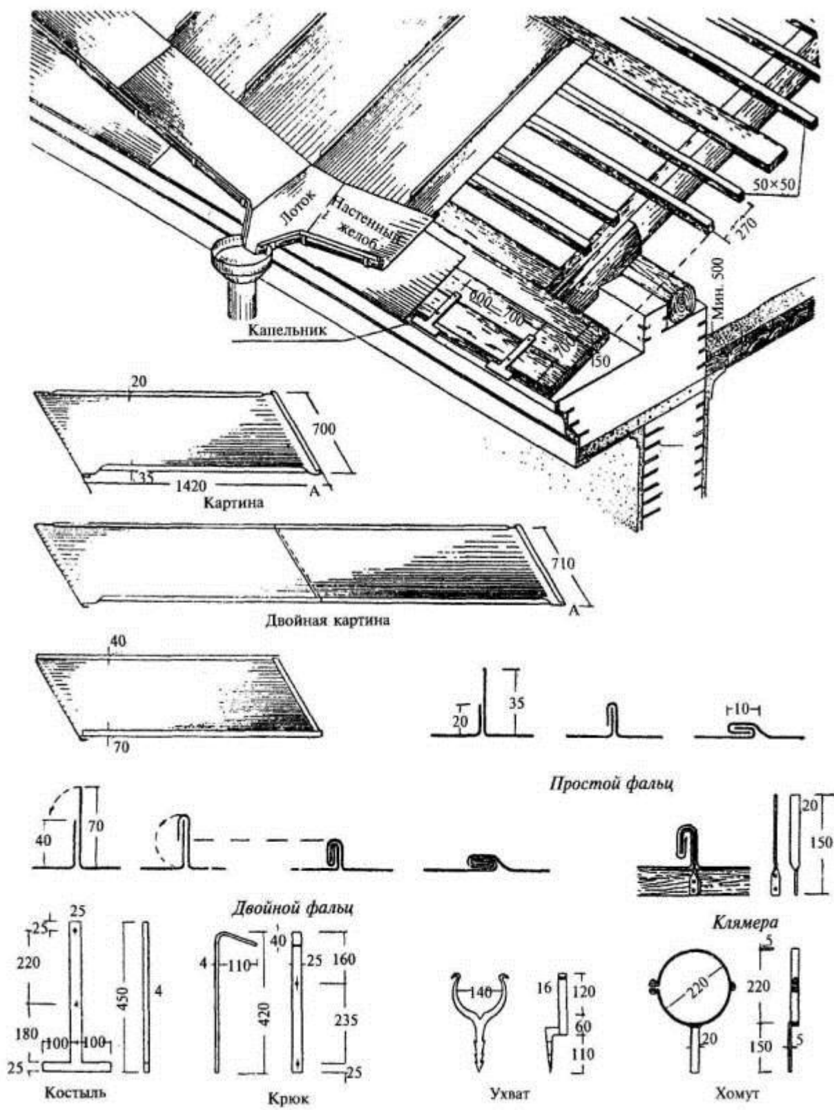
Детали железной кровли
