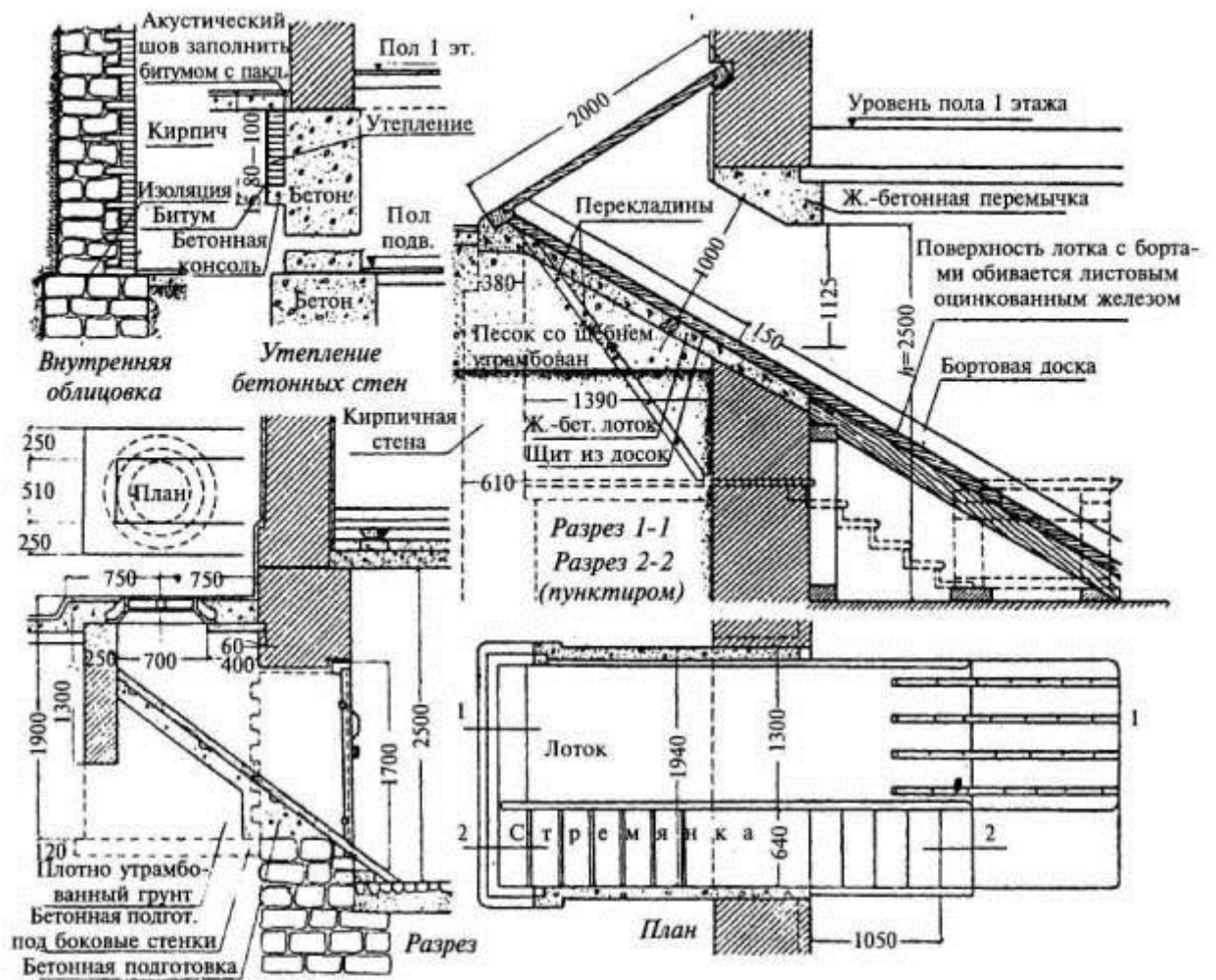
Люк для угля
