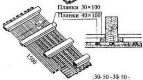
Накат из пустотелых камней (шлакобетон)
