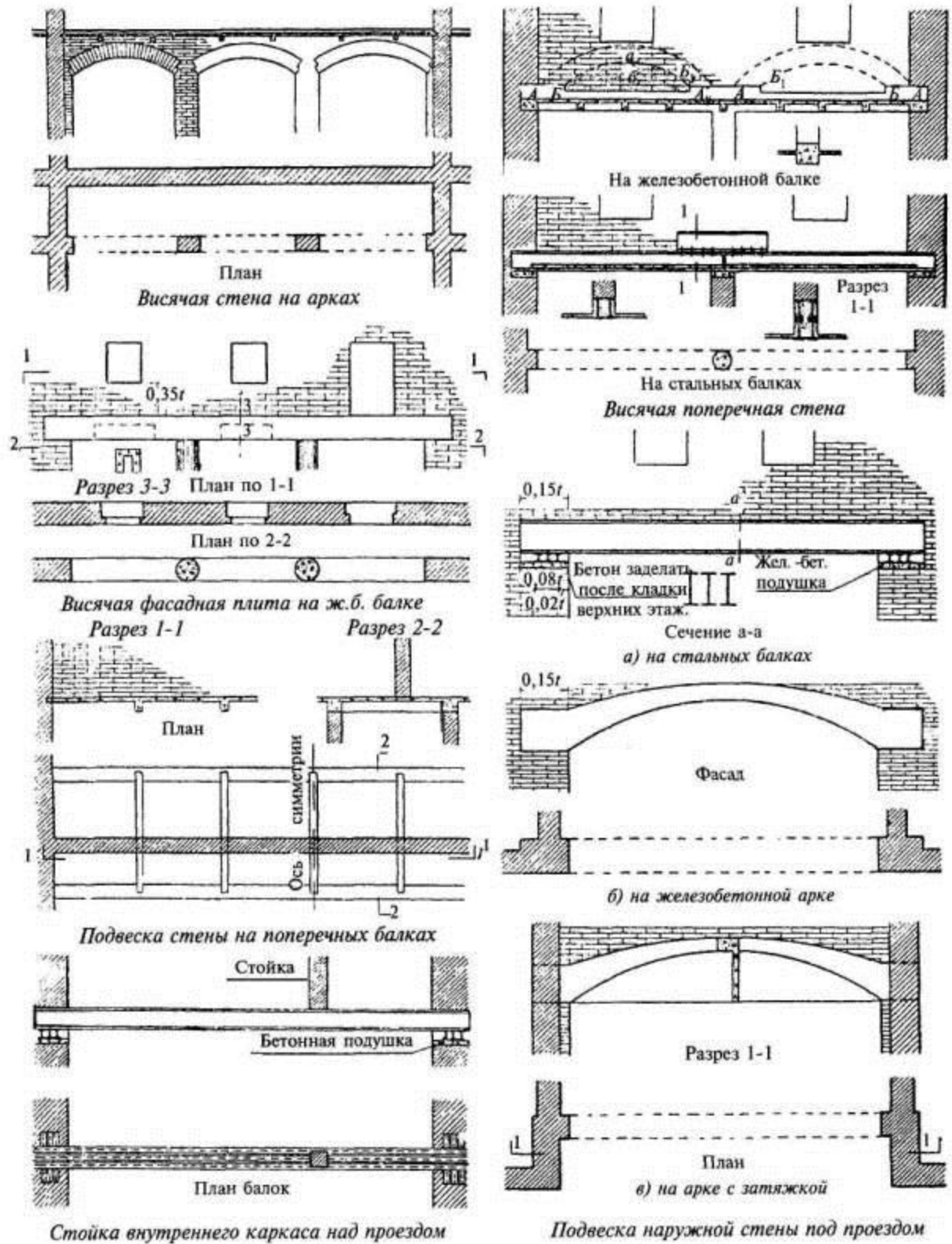
Местный каркас в массивных стенах
