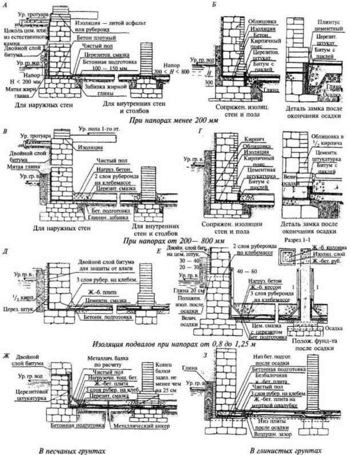
Защита подвалов от затопления водой
