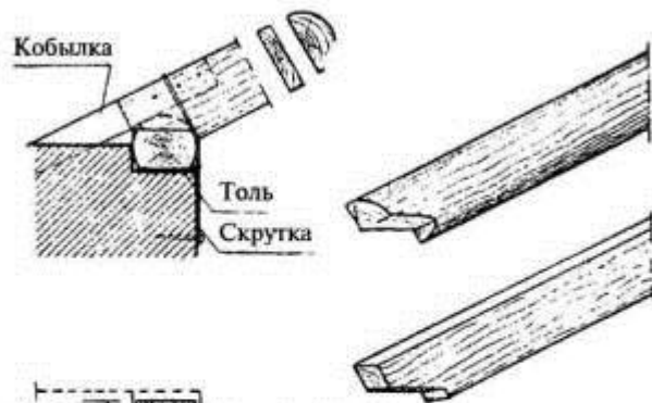
Опираие бревенчатой стропильной ноги на мауэрлат
