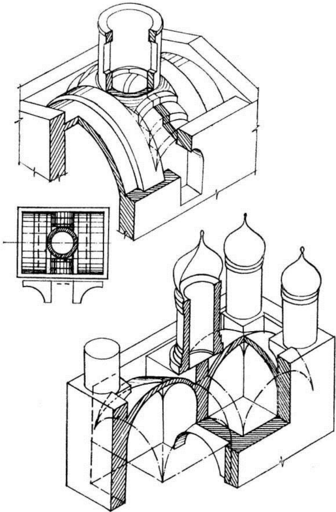
Бараны глав (схема Г. Б. Бессонова)
