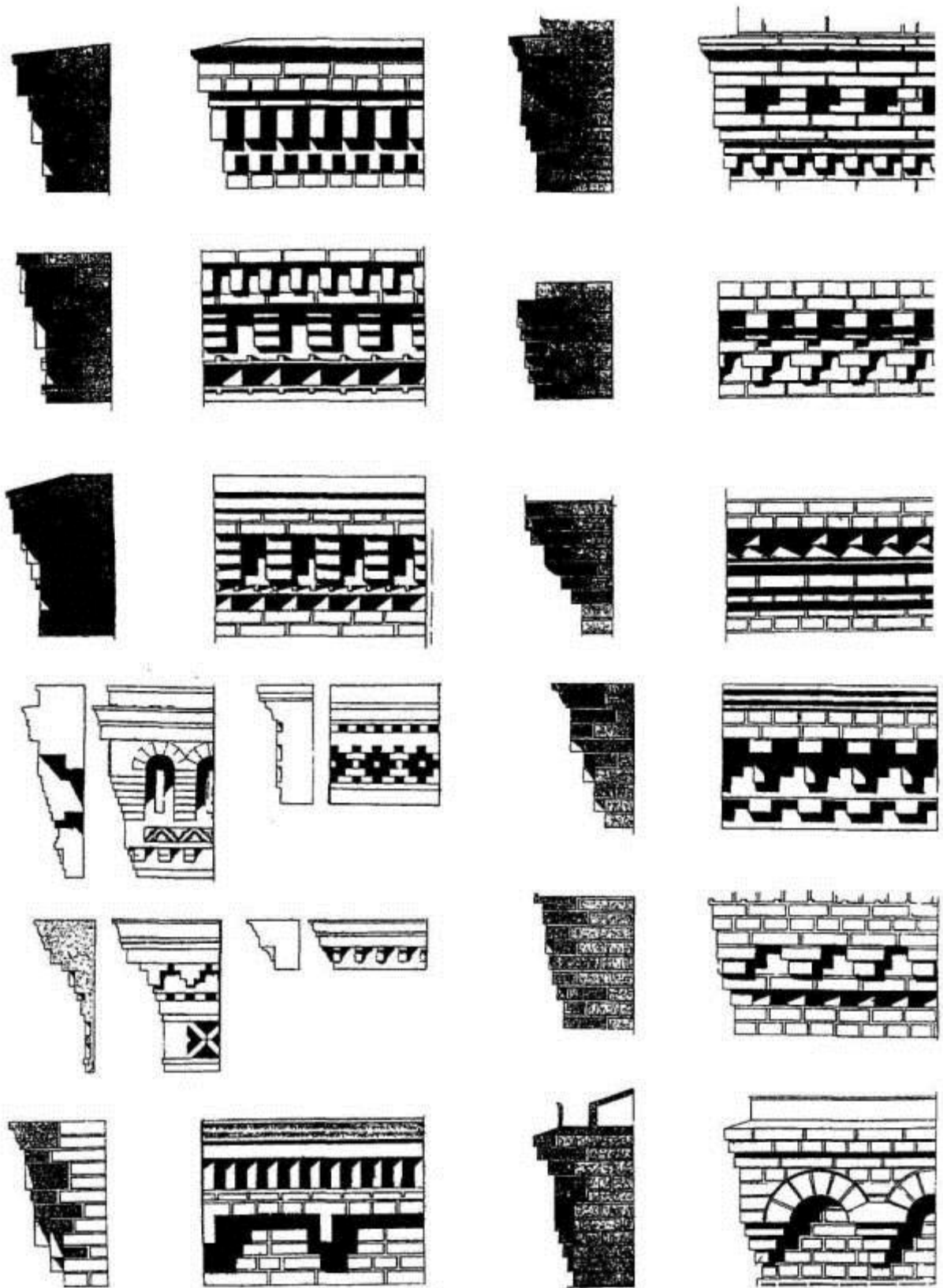
Карнизы из кирпича и камня
