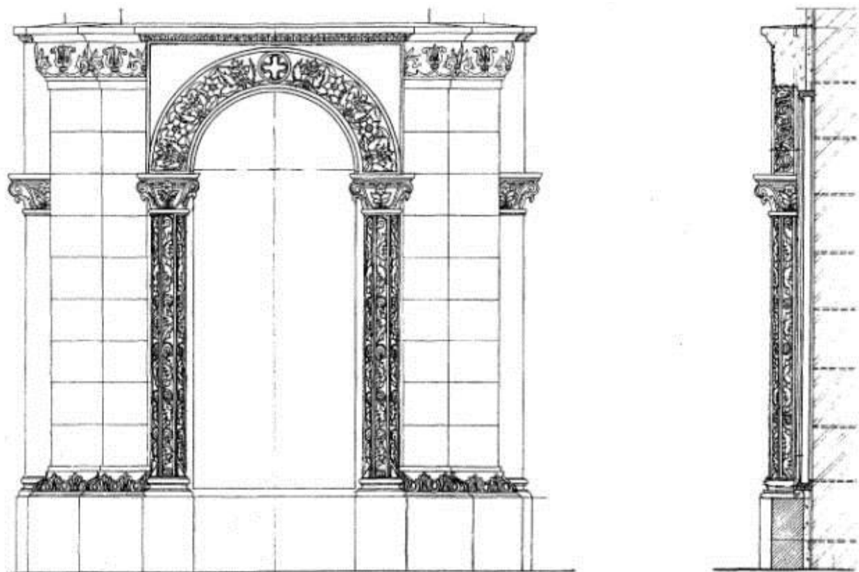
Белокаменный киот храма Преображения Господня в комплексе Храма Христа Спасителя (АХЦ «Арххрам»)
