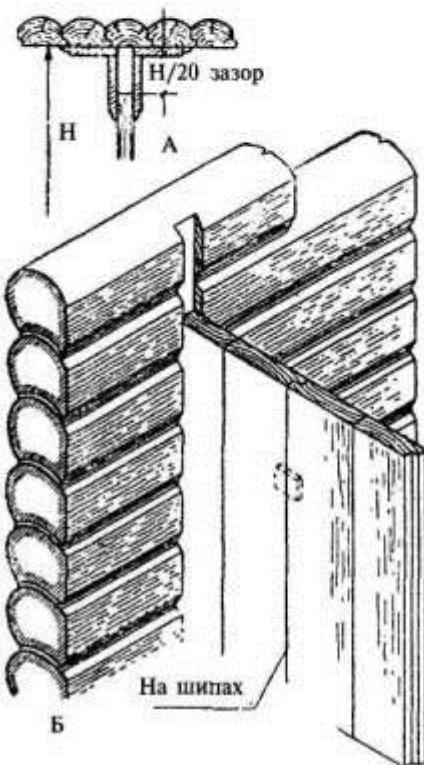
Присоединение перегородки к потолку (А) и к стене (Б)
