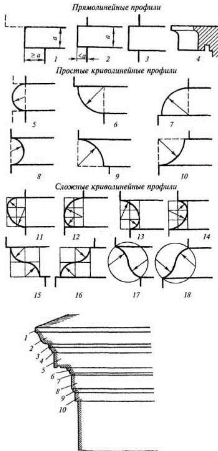
Архитектурные обломы
