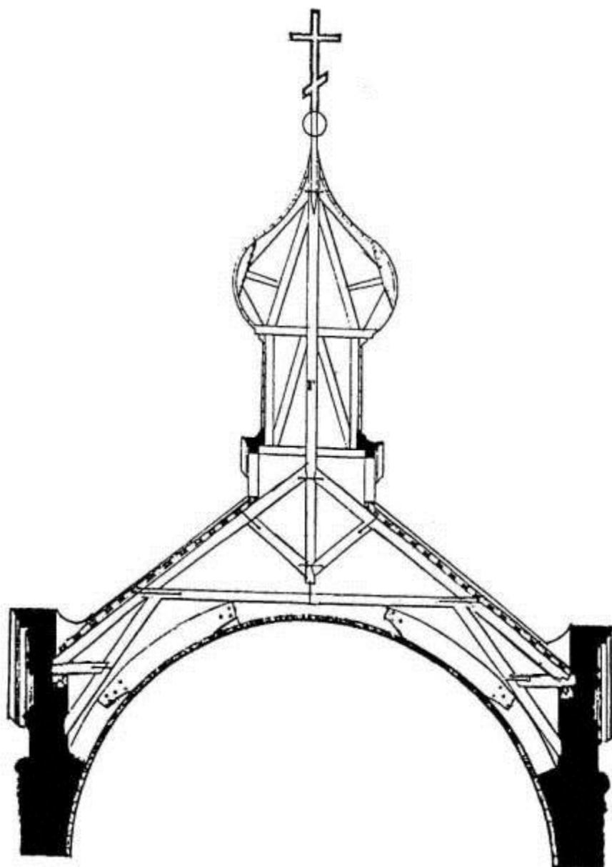
Конструкция деревянного покрытия храма (из атласа проектов храмов, 1911)
