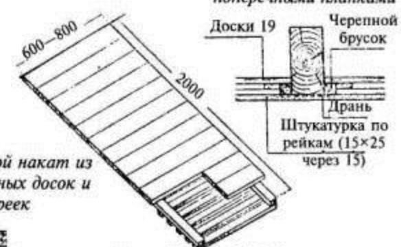
Щитовой накат из продольных досок с поперечными планками
