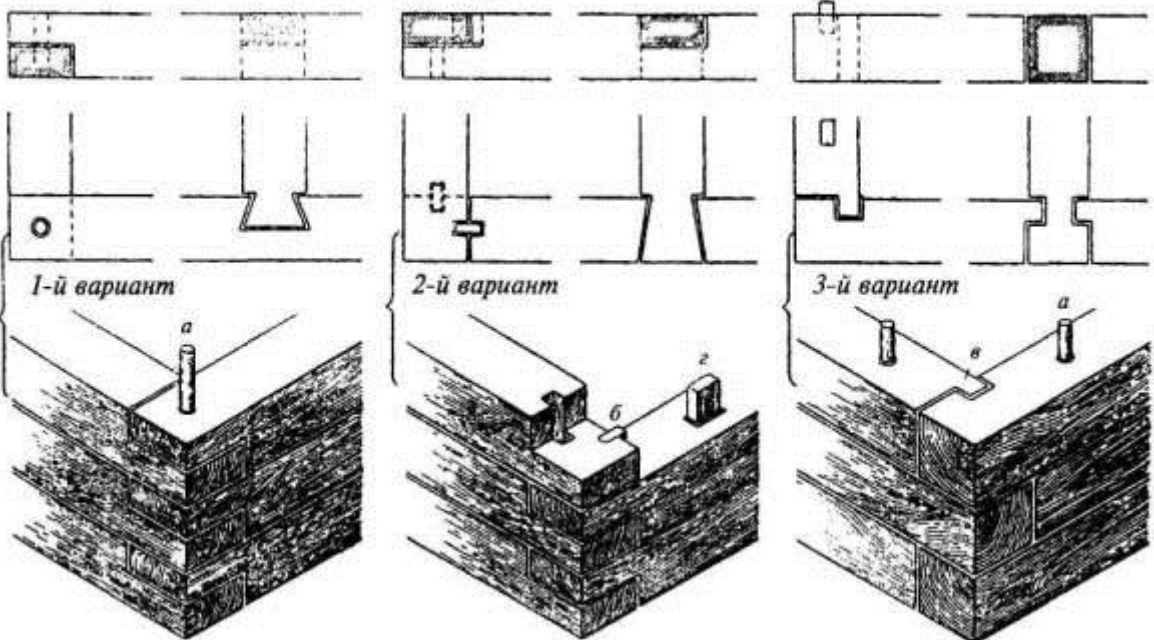
Сплачивание венцов из брусьев
