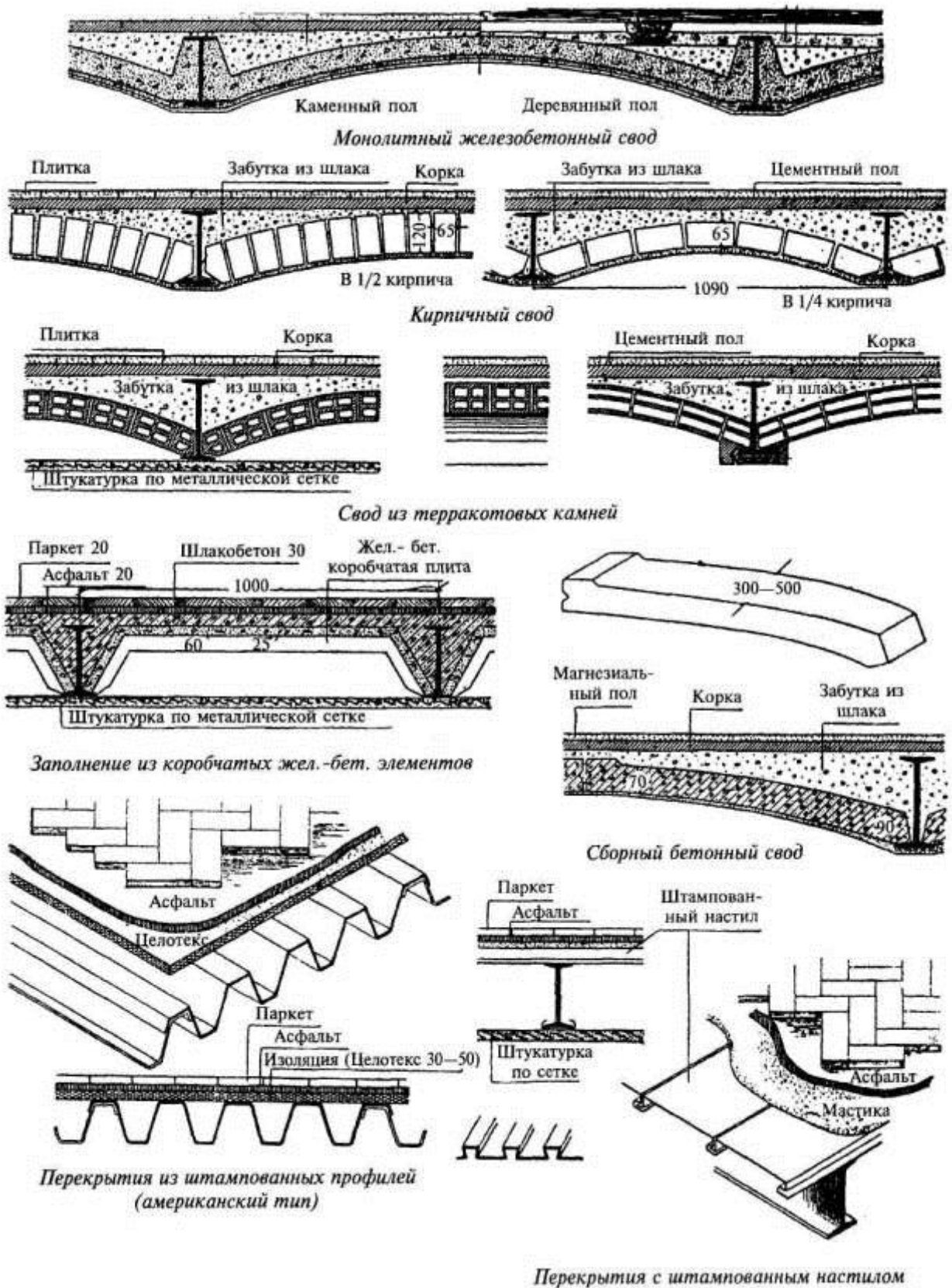
Перекрытия со стальными балками и сводчатым заполнением
