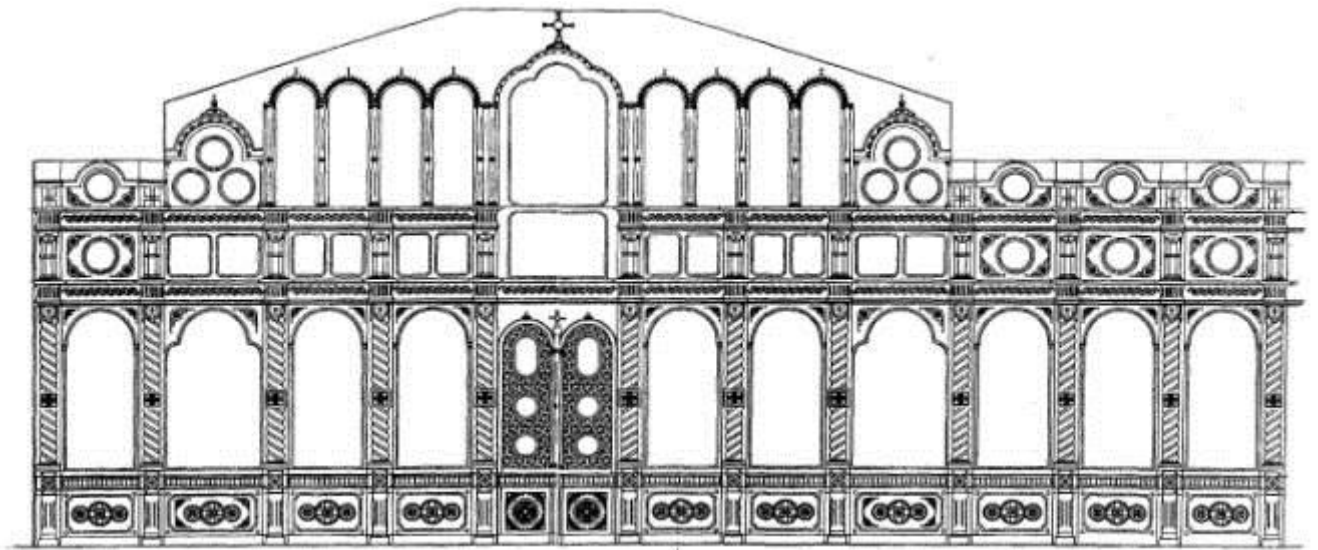
Проект иконостаса придела Преп, Серафима Сарюжкаш в Троицком храме в Удельной
