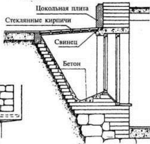
Приямок с наклонной кирпичной стенкой
