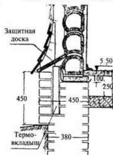
Цоколь с термо-вкладышем
