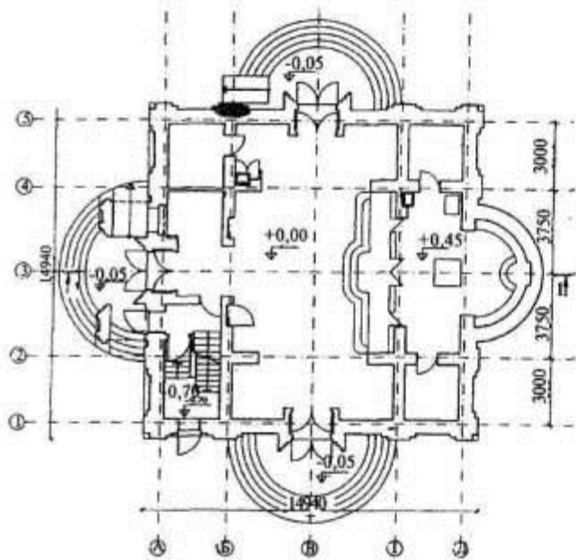
Храм в честь преподобномученицы Елизаветы в пос. Опалиха Красногорского р-на Московской области (АХЦ «Арххрам»)
