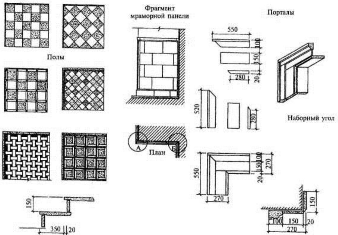
Элементы облицовки мрамором
