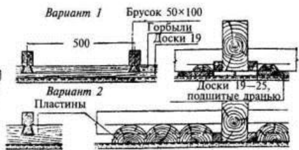
Щитовой накат из продольных пластин или горбылей
