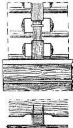
Детали обшивки рубленых стен
