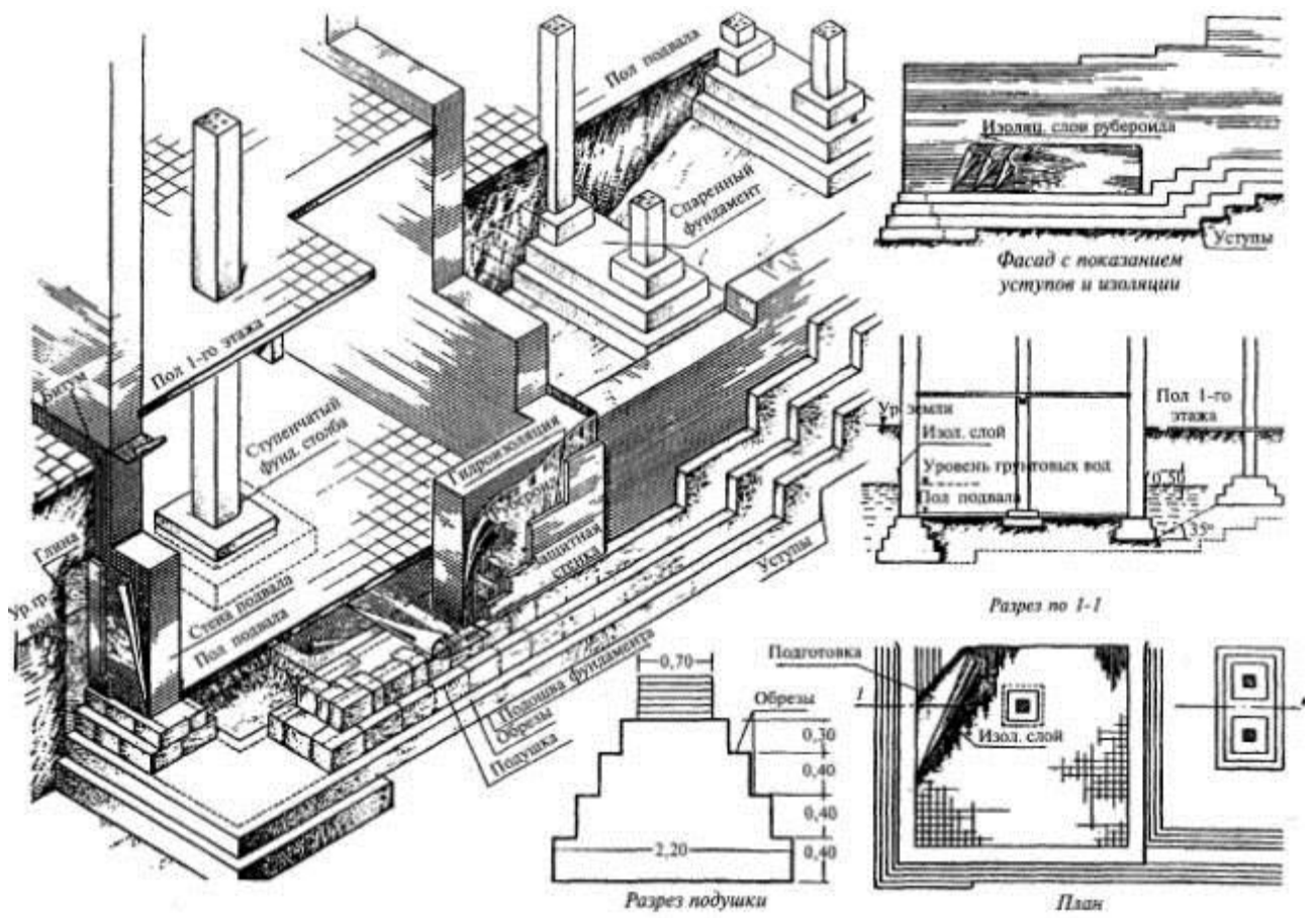
Общий вид фундаментов
