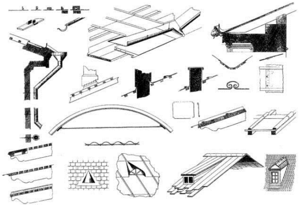
Кровли (из альбома А. Красовского, 1854)
