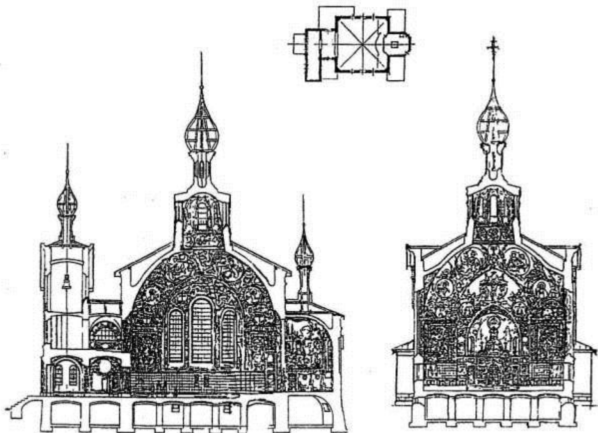
В.А. Ильин, гражд. инж. Проект храма при гимназии в Павлограде (1905)
