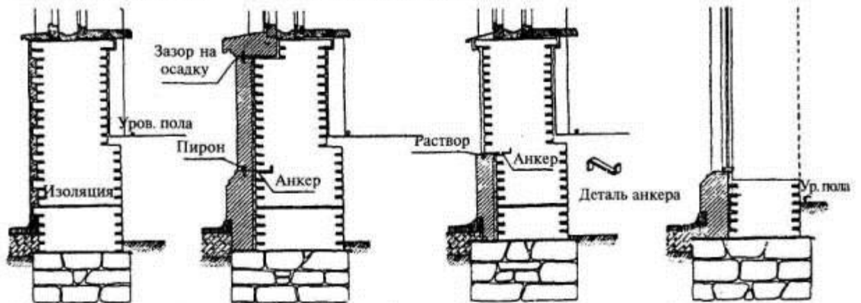
Цоколь, облицованный бетоном
