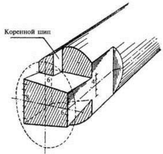
Лапа с коренным шипом 8×6×4 деления
