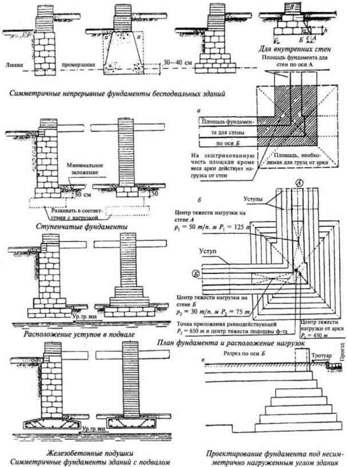
Фундаменты под массивными стенами
