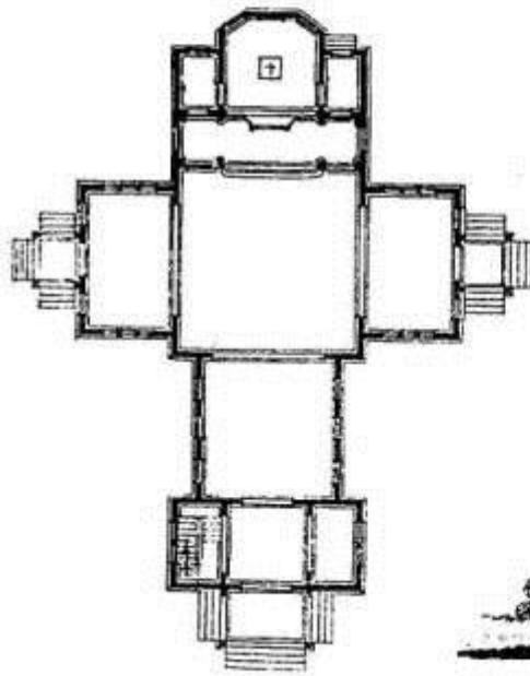
Проект деревянной церкви
