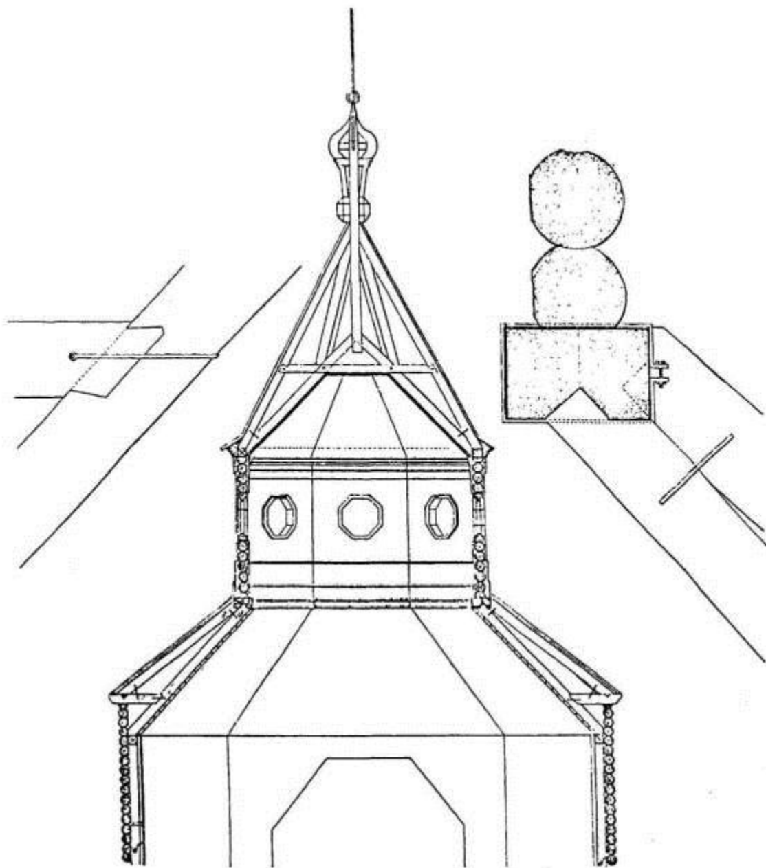
Шатровое завершение деревянного храма (из атласа проектов храмов, 1911)
