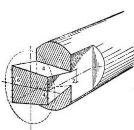
Простая лапа 6×4×2 деления
