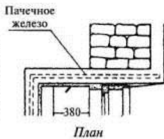
Малый приямок с кирпичными стенками
