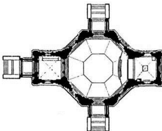
Проект каменной церкви на 400-500 чел. (1899)
