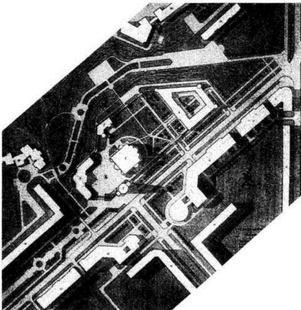
Храмовый комплекс. Духовный центр православия Республики Коми в городе Сыктывкаре
