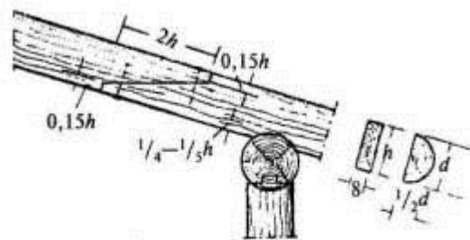
Прирубка дощатой стропильной ноги и стык на консоли
