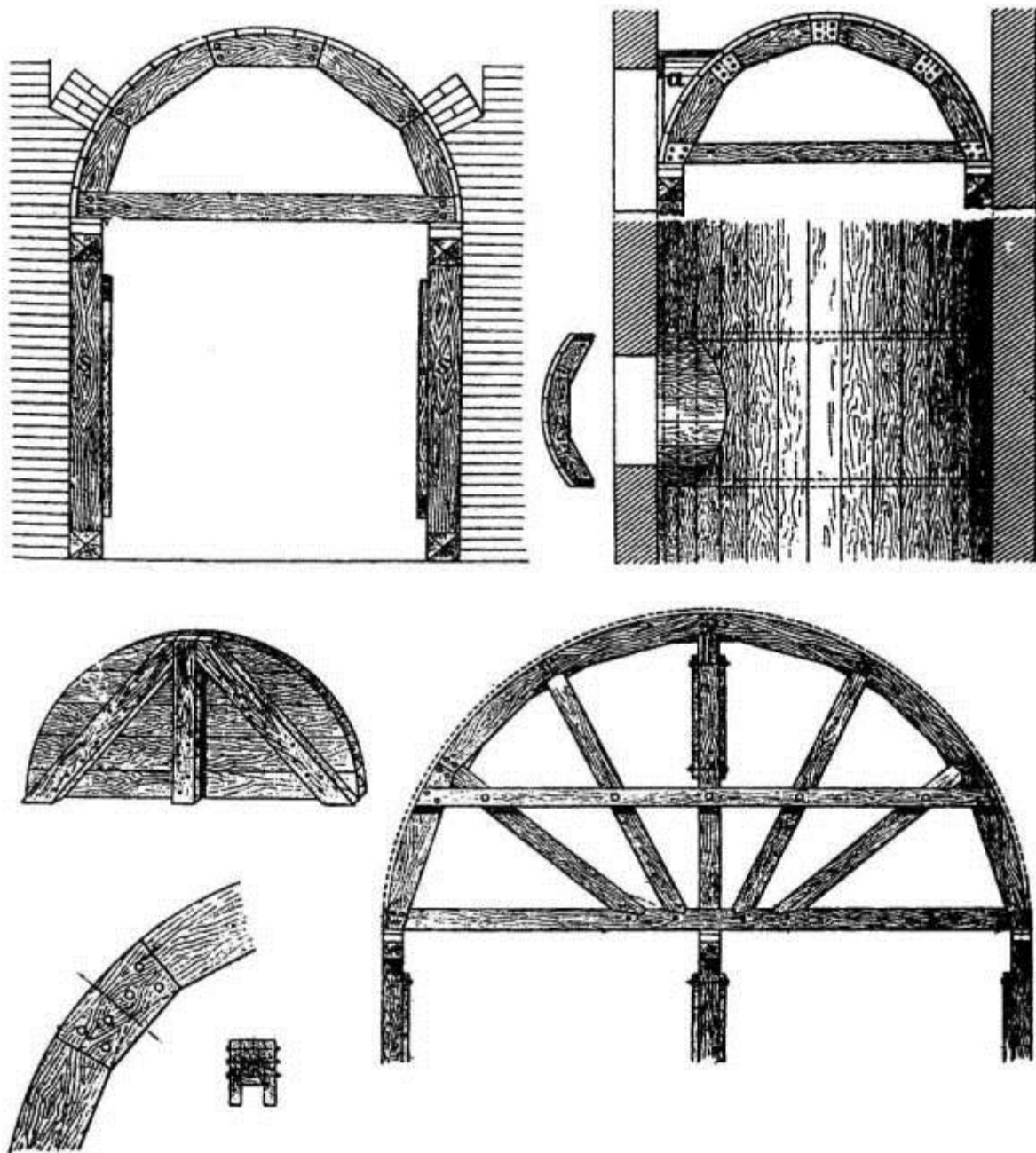
Арки и своды (из Руководства В. Р. Бернгарда, 1901)
