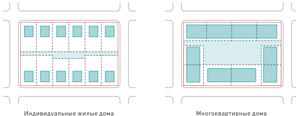
Илл. 54. Примеры межевания с выделением двора в отдельный земельный участок при застройке различными типами жилых домов
