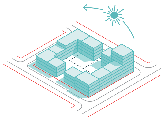
е) уточнение пространственного конверта с учетом требований инсоляции
